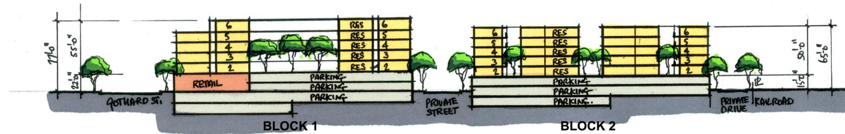
SECTION A-A
