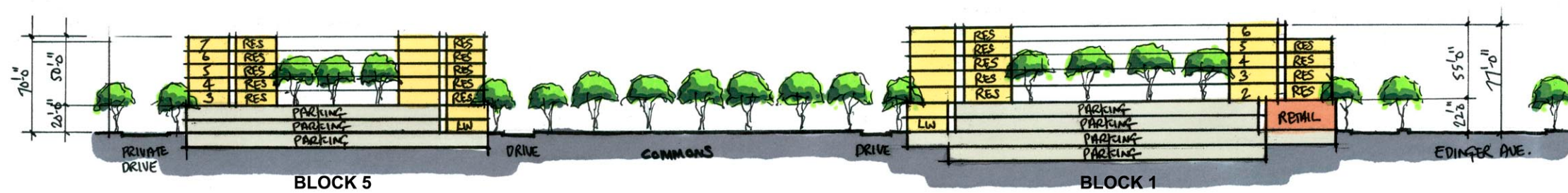
SECTION D-D
